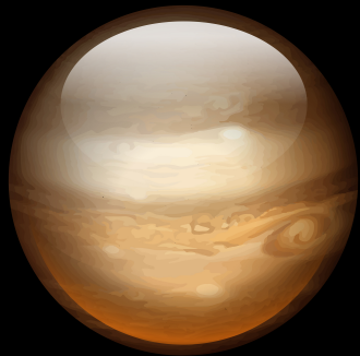
Planet Jupiter
