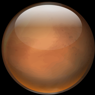
Planet Mars
