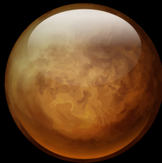
Planet Venus
