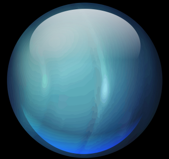
Planet Uranus
